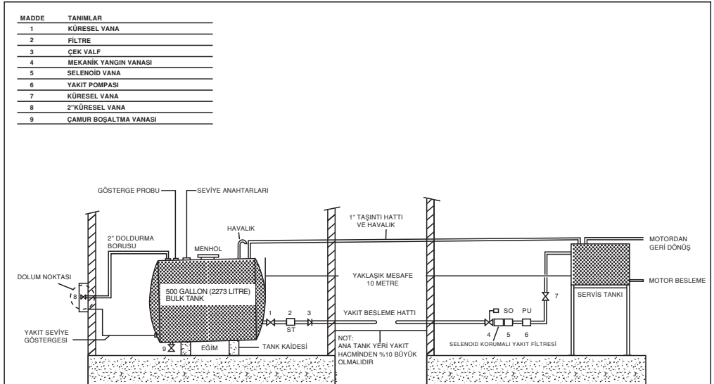
Şekil 4.3. Jeneratör grubu günlük servis yakıt tankı ve ana yakıt tankı için tipik bağlantı tesisi
