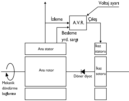
Şekil 11.1. Alternatör çalışması blok şeması
